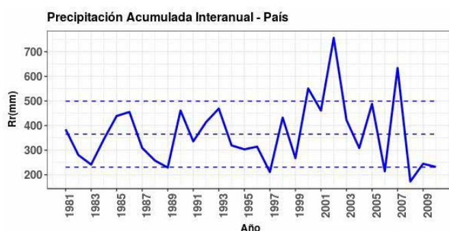
Fig.8: Precipitación acumulada interanual . La línea discontinua central de color azul representa el comportamiento medio, mientras que las restantes cuantifican la variabilidad mediante una desviación estándar.
