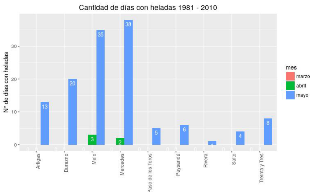
Fig.14: Cantidad de días con heladas por estación en MAM 1981 -2010
