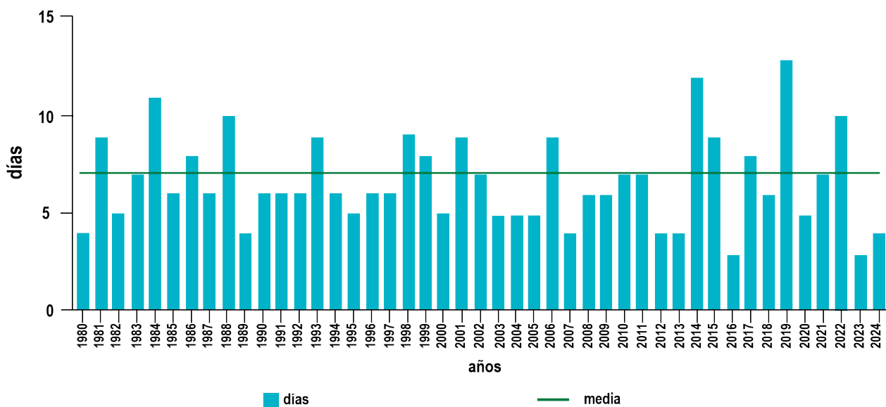
Figura 4: Cantidad de días con precipitación mayor o igual a 1.0 mm de los meses de febrero a escala país.
