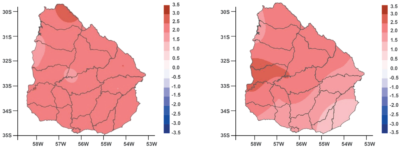
Figura 14: Mapa de anomalías de temperatura máxima media (a la izquierda) y de temperatura mínima media (a la derecha).
