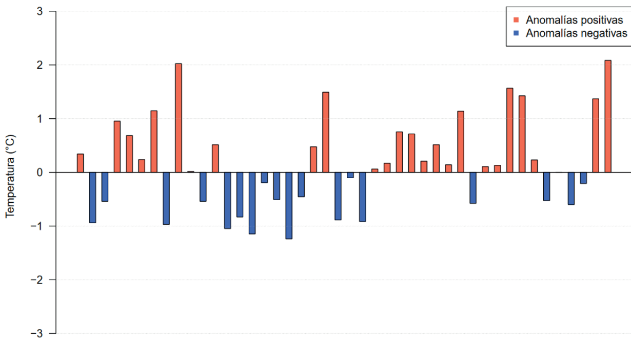
Figura 11: Anomalías de temperatura media a nivel país para los meses de febrero de 1981 a 2024.
