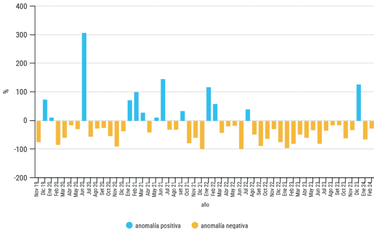
Figura 6: Evolución de anomalías mensuales de precipitación para la localidad de San Antonio.
