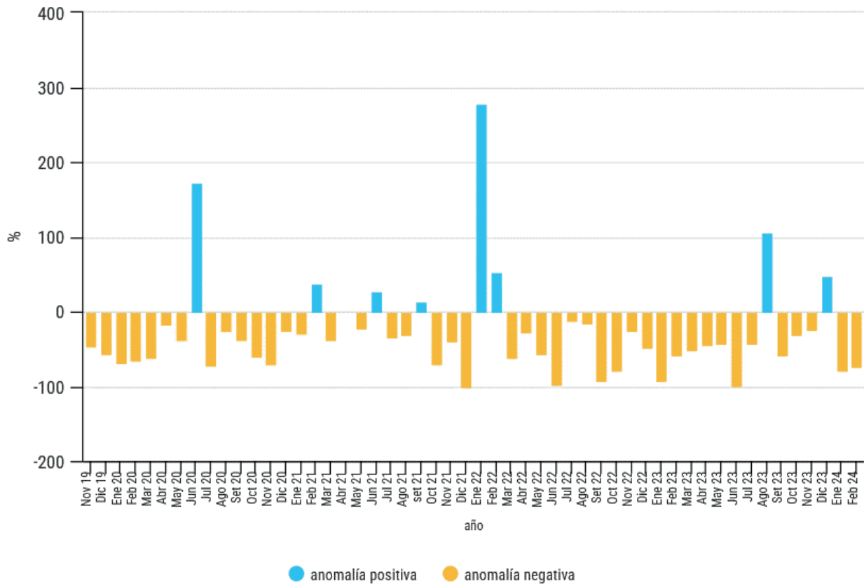
Figura 5: Evolución de anomalías mensuales de precipitación para la estación de Carrasco.
