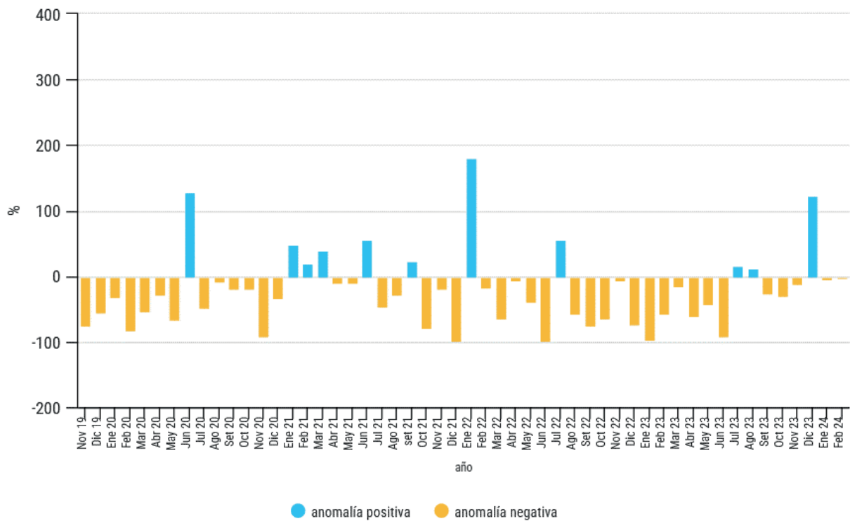
Figura 8: Evolución de anomalías mensuales de precipitación para la localidad de Tala.
