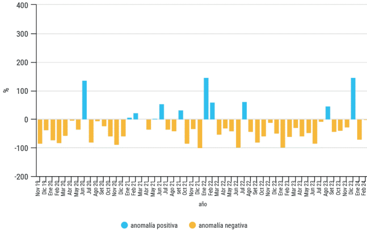
Figura 7: Evolución de anomalías mensuales de precipitación para la localidad de San Jacinto.
