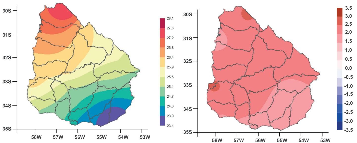
Figura 10: Mapa de temperatura media (izquierda) y anomalías de temperatura media (derecha) para febrero de 2024.
