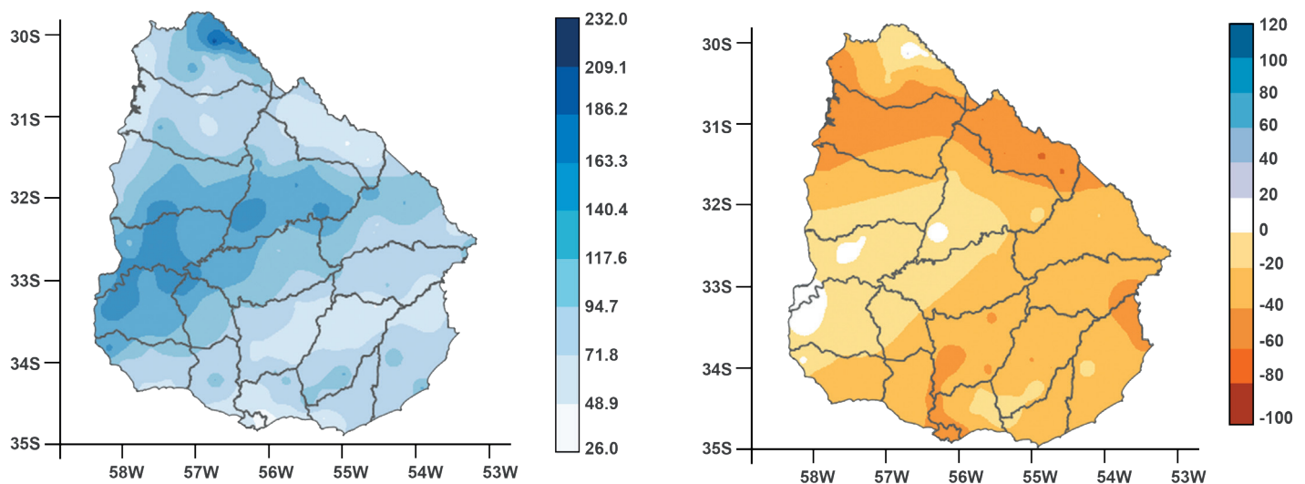
Figura 1: Mapa de precipitación acumulada en mm (izquierda) y anomalías de precipitación en porcentaje (derecha) para el mes de febrero de 2024.
