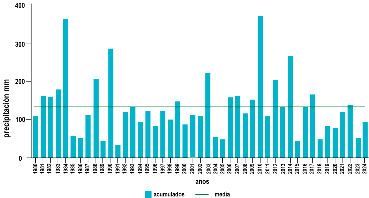
Figura 3: Precipitación acumulada promedio de los meses de febrero a escala país.
