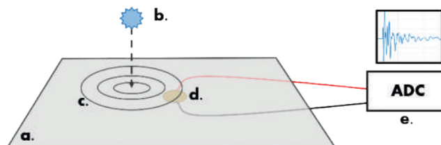
Figura 3 – Módulo del sensor de granizo.
