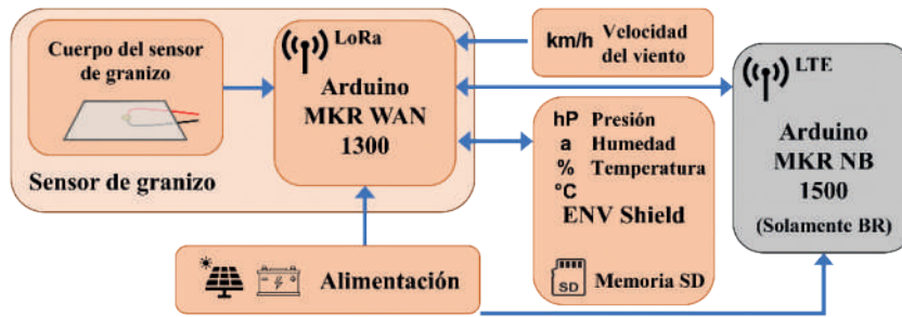
Figura 2 – Nodo de la red.
