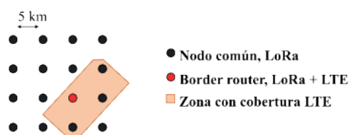
Figura 1 – Red de sensores.
