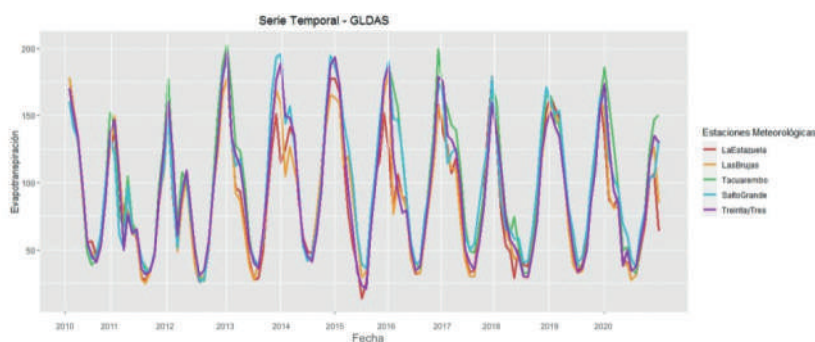
Figura 2. Serie temporal de las 5 localizaciones en el período 2010-2020 por la base de datos otorgada por GLDAS.
