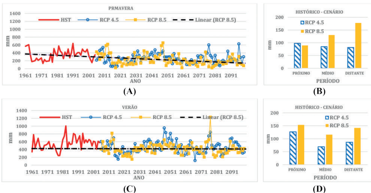
Figura 1 – Climatologia (histórico – HST) e projeção da variabilidade sazonal da precipitação total para diferentes cenários RCP 4,5 e RCP 8,5 (A e C), diferença entre a média da climatologia histórica (HST) e a média dos períodos próximo (2011 - 2040), médio (2041 - 2070) e distante (2071 - 2100) (B e D) e tendência (linha tracejada) para a região metropolitana de Goiânia (RMG) – Goiás.
