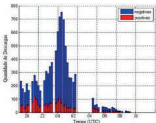
Figura 2 – Distribuição temporal, resolução 10 minutos, das descargas pelo sistema em estudo.
