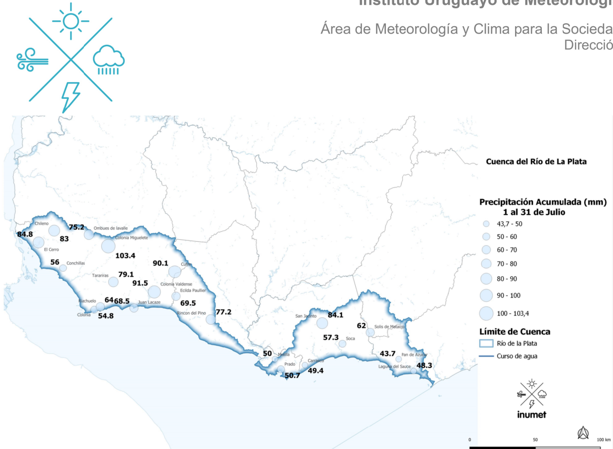
Figura 4 - Acumulados de precipitación del 1 al 31 de julio en la cuenca del Río de la Plata.
