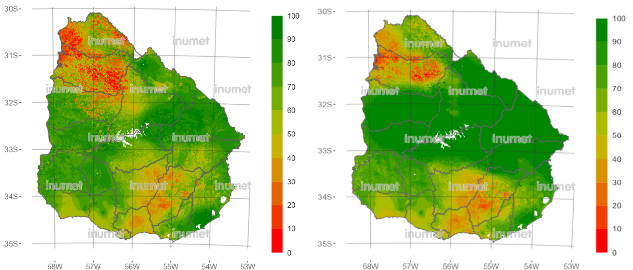
Figura 2 - Porcentaje de agua disponible en el suelo (%) del 11 al 20 (izq) y del 21 al 30 de junio de 2023 (der)
