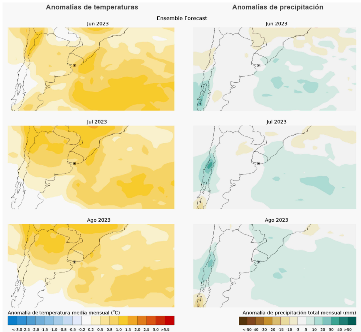
Figura 5 - Pronóstico climático mensual de anomalías de temperatura (izq) y de precipitación (der).
